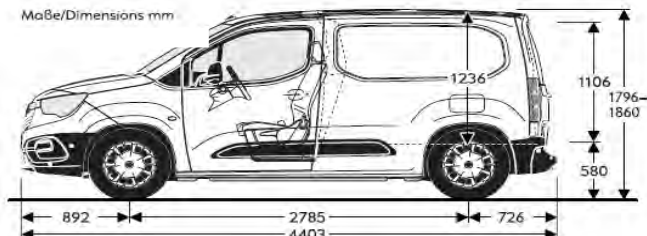
Maße/Dimensions mm
