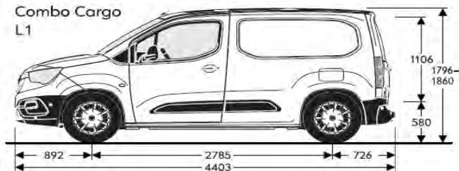
Maße/Dimensions mm
