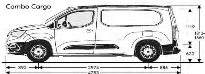
Maße/Dimensions mm
